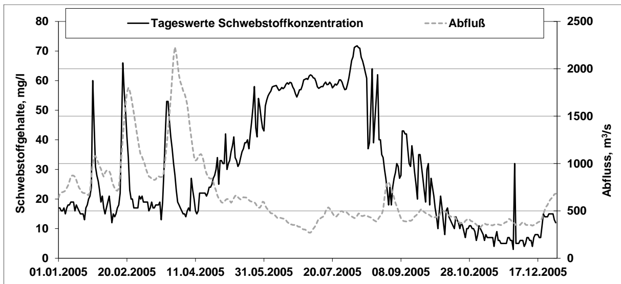
Abbildung 6: Jahrgang des Abflusses und der Schwebstoffgehalte am Pegel Wittenberge, Elbe-km 454,6, BfG.
