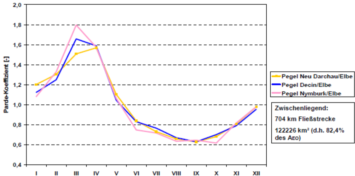
Abbildung 3: Abflussregime der Elbe an drei repräsentativen Pegeln. Methode nach Pardé, Bezugsperiode 1901(1931)-2010 (aus Belz 2013).
