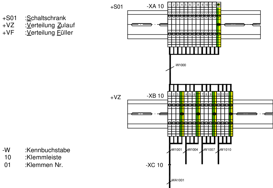
Abb. 6.6: Beispiel Kabelbeschriftung
