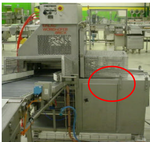
Abb. 6.2: Vorderansicht Beutelfüllgerät
