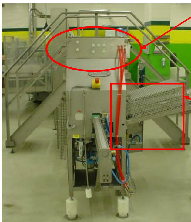
Abb. 6.1: Seitenansicht Beutelfüllgerät
